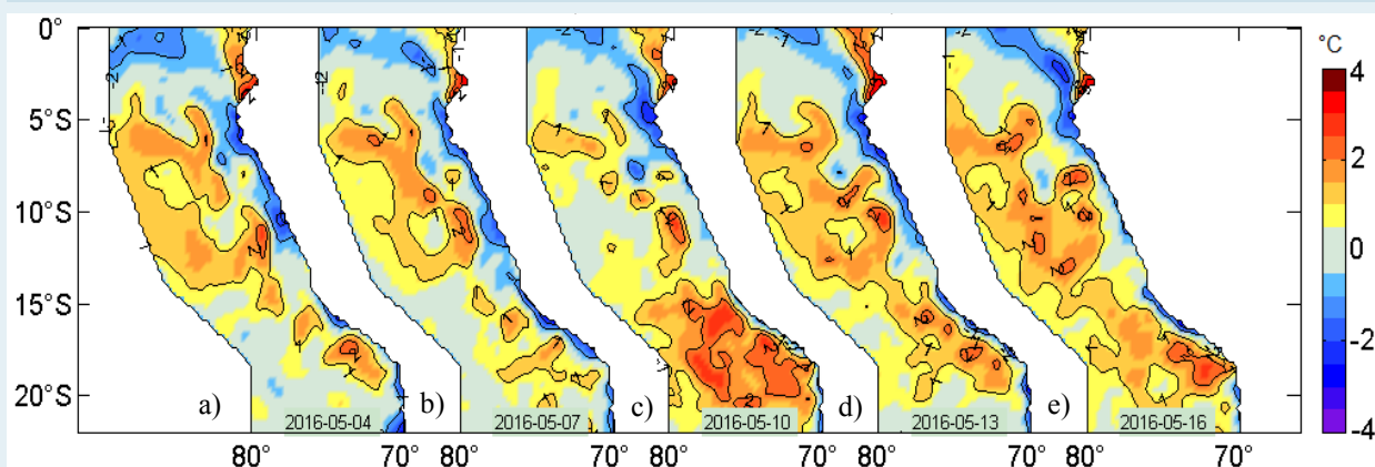
Figura 2. Anomalías de la temperatura superficial del agua (°C) en el mar peruano, cada tres días, entre el 04 y 16 de mayo del 2016. Datos: AVHRR Global Reyn_SmithOiv2R (Reynolds, et. al., 2007) de CMB/EMC/NCEP de la Administración Nacional del Océano y la Atmósfera (NOAA, según sus siglas en inglés). Procesamiento: IMARPE.
