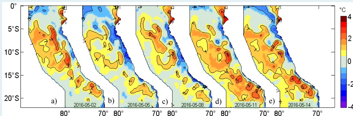
Figura 2. Anomalías de la temperatura superficial del agua (°C) en el mar peruano, cada tres días, entre el 02 y 14 de mayo del 2016. Datos: AVHRR Global Reyn_SmithOiv2R (Reynolds, et. al., 2007) de CMB/EMC/NCEP de la Administración Nacional del Océano y la Atmósfera (NOAA, según sus siglas en inglés). Procesamiento: IMARPE.
