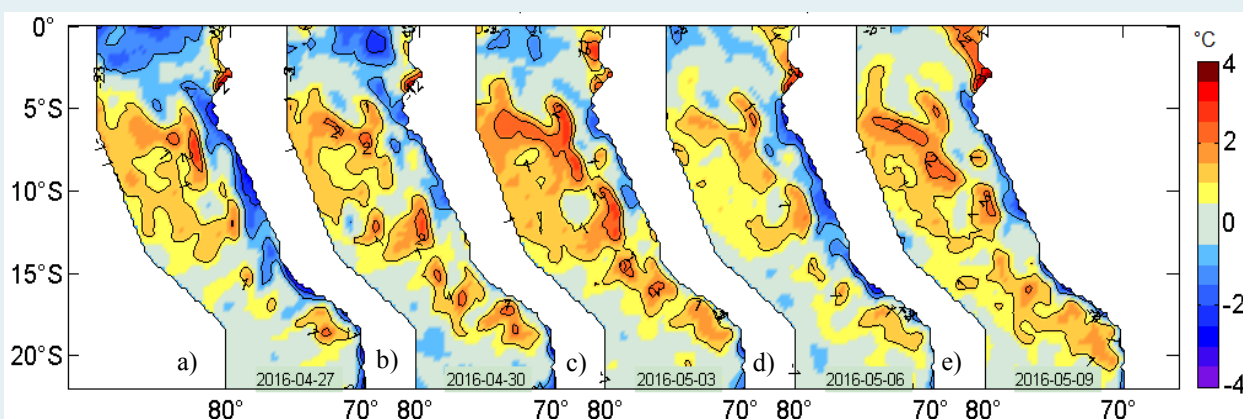
Figura 2. Anomalías de la temperatura superficial del agua (°C) en el mar peruano, cada tres días, entre el 27 de abril y 09 de mayo del 2016. Datos: AVHRR Global Reyn_SmithOlv2R (Reynolds, et. al., 2007) de CMB/EMC/NCEP de la NOAA. Procesamiento: IMARPE.
