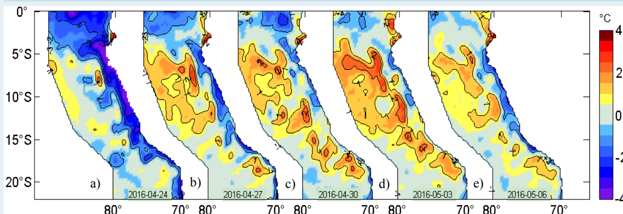
Figura 2. Anomalías de la temperatura superficial del agua (°C) en el mar peruano, cada tres días, entre el 24 de abril y 06 de mayo del 2016. Datos: AVHRR Global Reyn_SmithOiv2R (Reynolds, et. al., 2007) de CMB/EMC/NCEP de la Administración Nacional del Océano y la Atmósfera (NOAA, según sus siglas en inglés). Procesamiento: IMARPE.
