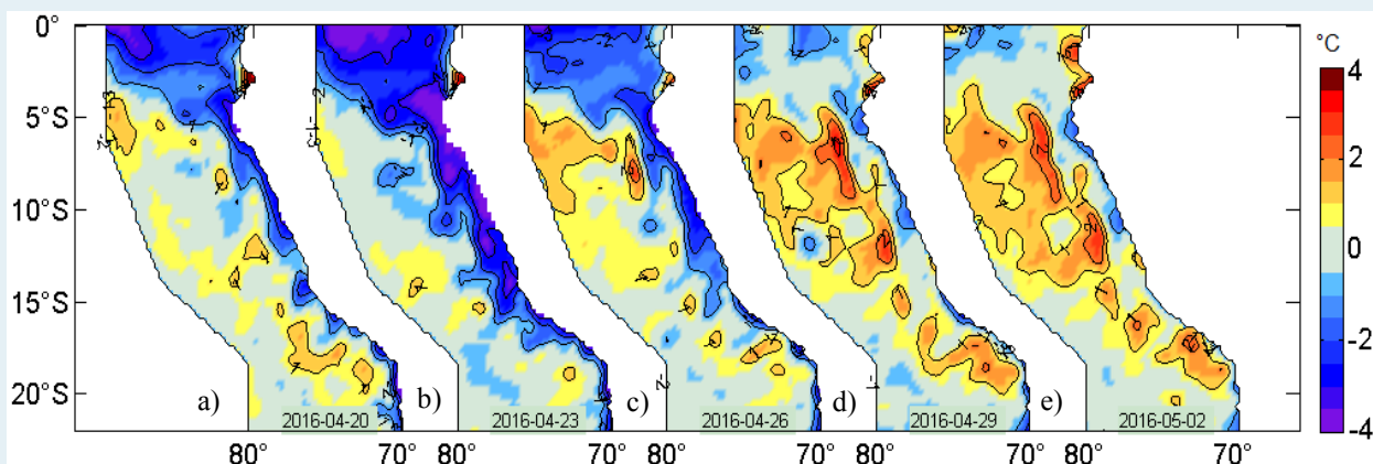
Figura 2. Anomalías de la temperatura superficial del agua (°C) en el mar peruano, cada tres días, entre el 20 de abril y 02 de mayo del 2016. Datos: AVHRR Global Reyn_SmithOiv2R (Reynolds, et. al., 2007) de CMB/EMC/NCEP de la Administración Nacional del Océano y la Atmósfera (NOAA, según sus siglas en inglés). Procesamiento: IMARPE.
