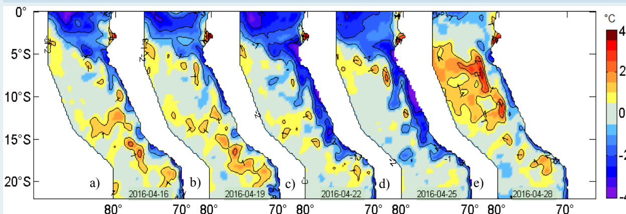
Figura 2. Anomalías de la temperatura superficial del agua (°C) en el mar peruano, cada tres días, entre el 16 y 28 de abril del 2016. Datos: AVHRR Global Reyn_SmithOlv2R (Reynolds, et. al., 2007) de CMB/EMC/NCEP de la Administración Nacional del Océano y la Atmósfera (NOAA, según sus siglas en inglés). Procesamiento: IMARPE.
