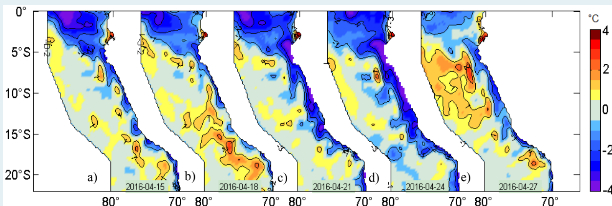
Figura 2. Anomalías de la temperatura superficial del agua (°C) en el mar peruano, cada tres días, entre el 15 y 27 de abril del 2016. Datos: AVHRR Global Reyn_SmithOiv2R (Reynolds, et. al., 2007) de CMB/EMC/NCEP de la Administración Nacional del Océano y la Atmósfera (NOAA, según sus siglas en inglés). Procesamiento: IMARPE.
