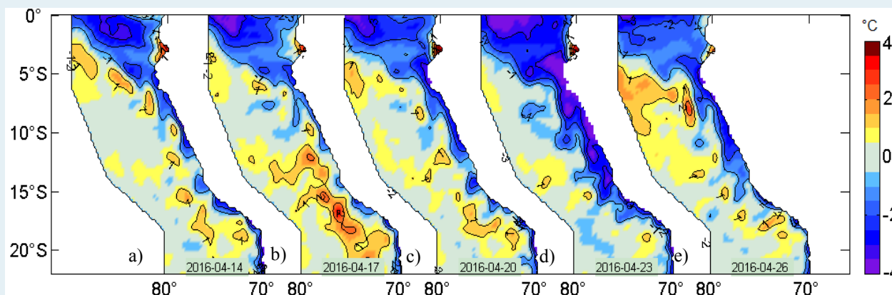
Figura 2. Anomalías de la temperatura superficial del agua (°C) en el mar peruano, cada tres días, entre el 14 y 26 de abril del 2016. Datos: AVHRR Global Reyn_SmithOiv2R (Reynolds, et. al., 2007) de CMB/EMC/NCEP de la Administración Nacional del Océano y la Atmósfera (NOAA, según sus siglas en inglés). Procesamiento: IMARPE.
