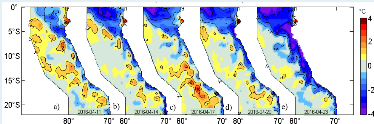
Figura 2. Anomalías de la temperatura superficial del agua (°C) en el mar peruano, cada tres días, entre el 11 y 23 de abril del 2016. Datos: AVHRR Global Reyn_SmithO1v2R (Reynolds, et. al., 2007) de CMB/EMC/NCEP de la Administración Nacional del Océano y la Atmósfera (NOAA, según sus siglas en inglés). Procesamiento: IMARPE.
