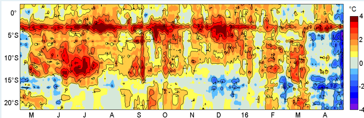
Figura 3. Evolución latitudinal de las anomalías promedio diarias de la temperatura superficial del mar (°C) para la franja de ~50 mn adyacentes al litoral peruano. Datos: AVHRR Global Reyn_SmithO1v2R (Reynolds, et. al., 2007) de CMB/EMC/NCEP de la Administración Nacional del Océano y la Atmósfera (NOAA, según sus siglas en inglés). Procesamiento: IMARPE.
