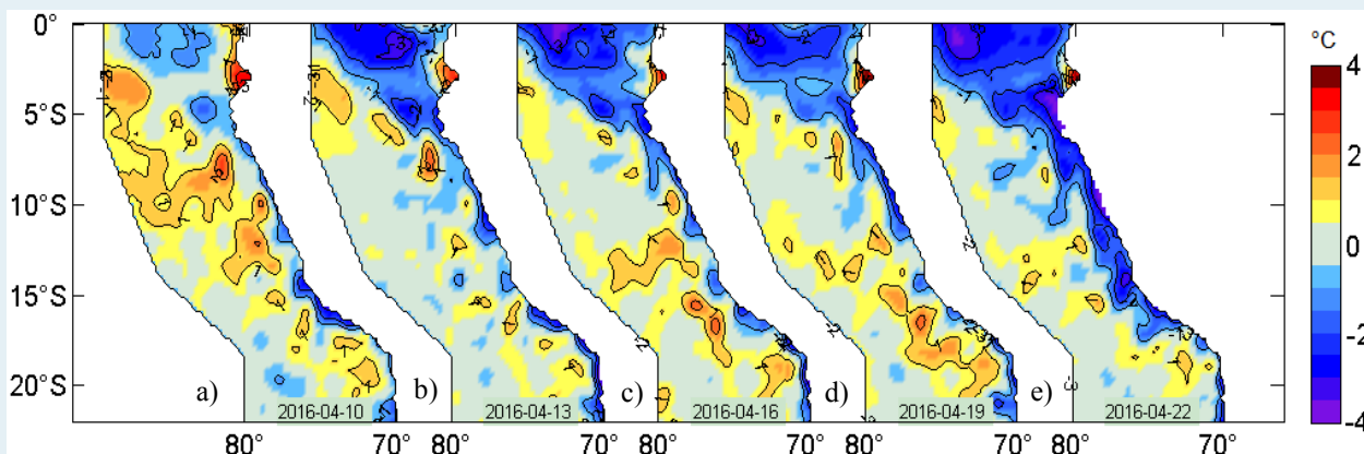
Figura 2. Anomalías de la temperatura superficial del agua (°C) en el mar peruano, cada tres días, entre el 10 y 22 de abril del 2016. Datos: AVHRR Global Reyn_SmithO1v2R (Reynolds, et. al., 2007) de CMB/EMC/NCEP de la Administración Nacional del Océano y la Atmósfera (NOAA, según sus siglas en inglés). Procesamiento: IMARPE.
