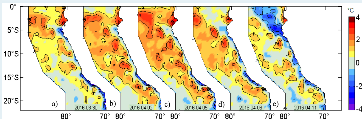
Figura 2. Anomalías de la temperatura superficial del agua (°C) en el mar peruano, cada tres días, entre el 30 de marzo y 11 de abril del 2016. Datos: AVHRR Global Reyn_SmithOlv2R (Reynolds, et. al., 2007) de CMB/EMC/NCEP de la Administración Nacional del Océano y la Atmósfera (NOAA, según sus siglas en inglés). Procesamiento: IMARPE.
