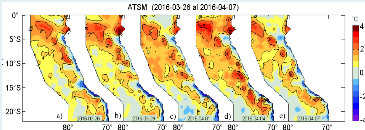
Figura 2. Anomalías de la temperatura superficial del agua (°C) en el mar peruano, cada tres días, entre el 26 de marzo y 07 de abril del 2016. Datos: AVHRR/NOAA. Procesamiento: IMARPE.
