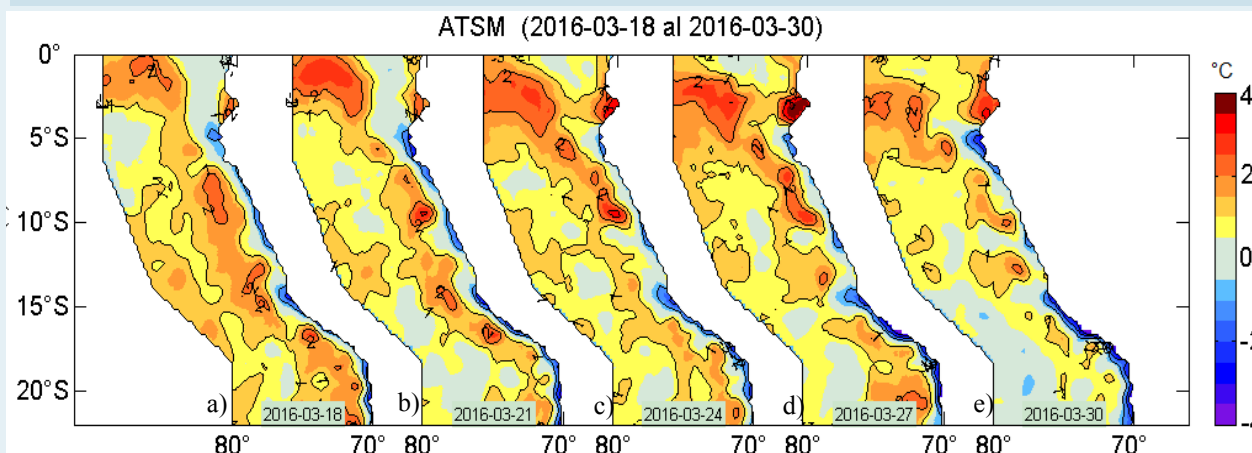
Figura 2. Anomalías de la temperatura superficial del agua (°C) en el mar peruano, cada tres días, entre el 18 y 30 de marzo del 2016. Datos: AVHRR/NOAA. Procesamiento: IMARPE.
