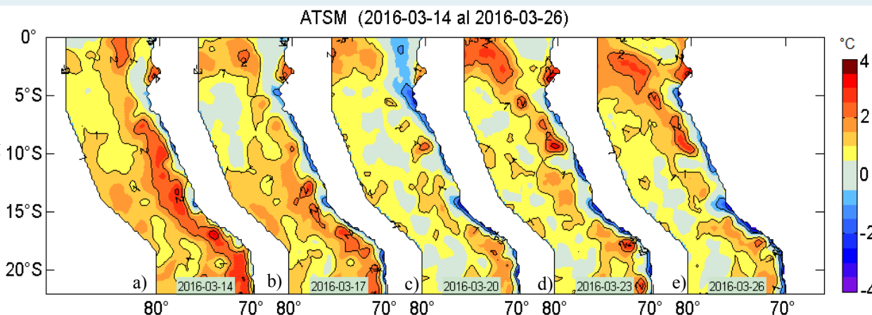
Figura 2. Anomalías de la temperatura superficial del agua (°C) en el mar peruano, cada tres días, entre el 14 y 26 de marzo del 2016. Datos: AVHRR de NOAA. Procesamiento: IMARPE.
