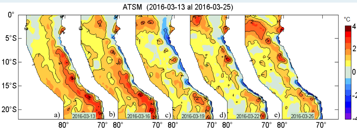
Figura 2. Anomalías de la temperatura superficial del agua (°C) en el mar peruano, cada tres días, entre el 13 y 25 de marzo del 2016. Datos: AVHRR de NOAA. Procesamiento: IMARPE.
