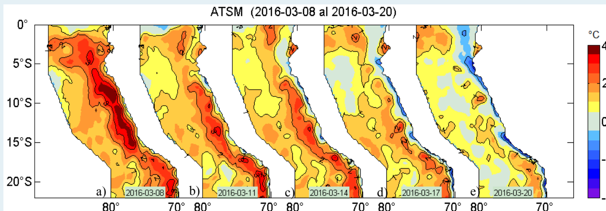
Figura 2. Anomalías de la temperatura superficial del agua (°C) en el mar peruano, cada tres días, entre el 08 y 20 de marzo del 2016. Datos: AVHRR de NOAA. Procesamiento: IMARPE.
