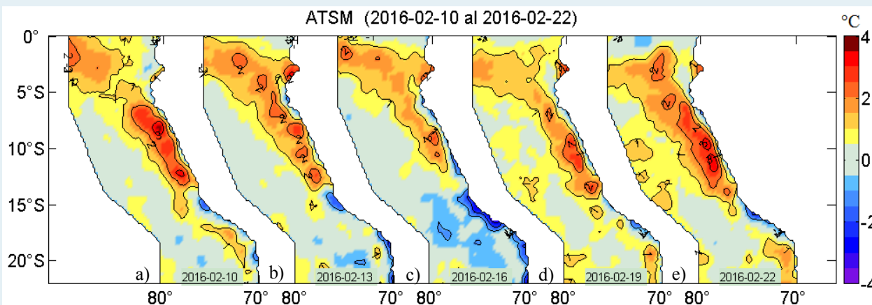
Figura 2. Anomalías de la temperatura superficial del agua (°C) en el mar peruano, cada tres días, entre el 10 y 22 de febrero del 2016. Datos: AVHRR de NOAA. Procesamiento: IMARPE.
