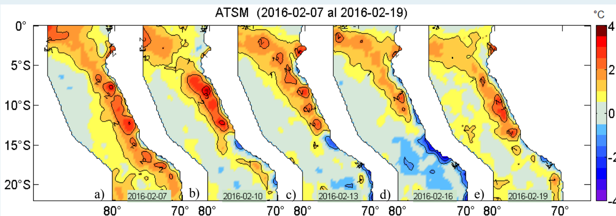
Figura 2. Anomalías de la temperatura superficial del agua (°C) en el mar peruano, cada tres días, entre el 07 al 19 de febrero del 2016. Datos: AVHRR/NOAA. Procesamiento: IMARPE.
