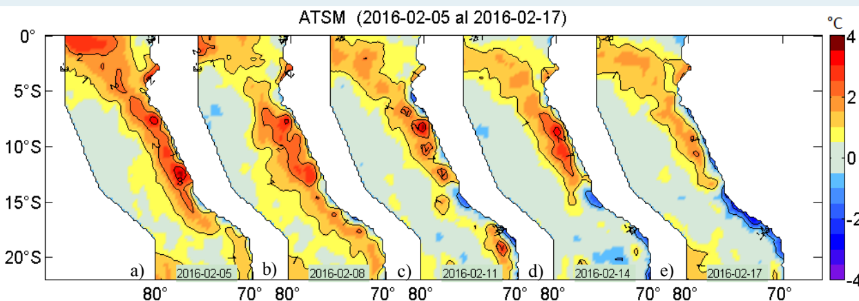
Figura 2. Anomalías de la temperatura superficial del agua (°C) en el mar peruano, cada tres días, entre el 05 al 17 de febrero del 2016. Datos: AVHRR de NOAA. Procesamiento: IMARPE.
