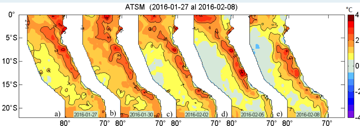
Figura 2. Anomalías de la temperatura superficial del agua (°C) en el mar peruano, cada tres días, entre el 27 de enero y 08 de febrero del 2016. Datos: AVHRR/NOAA. Procesamiento: IMARPE.
