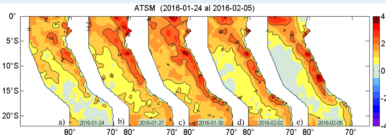
Figura 2. Anomalías de la temperatura superficial del agua (°C) en el mar peruano, cada tres días, entre el 24 de enero al 05 de febrero del 2016. Datos: AVHRR/NOAA. Procesamiento: IMARPE.
