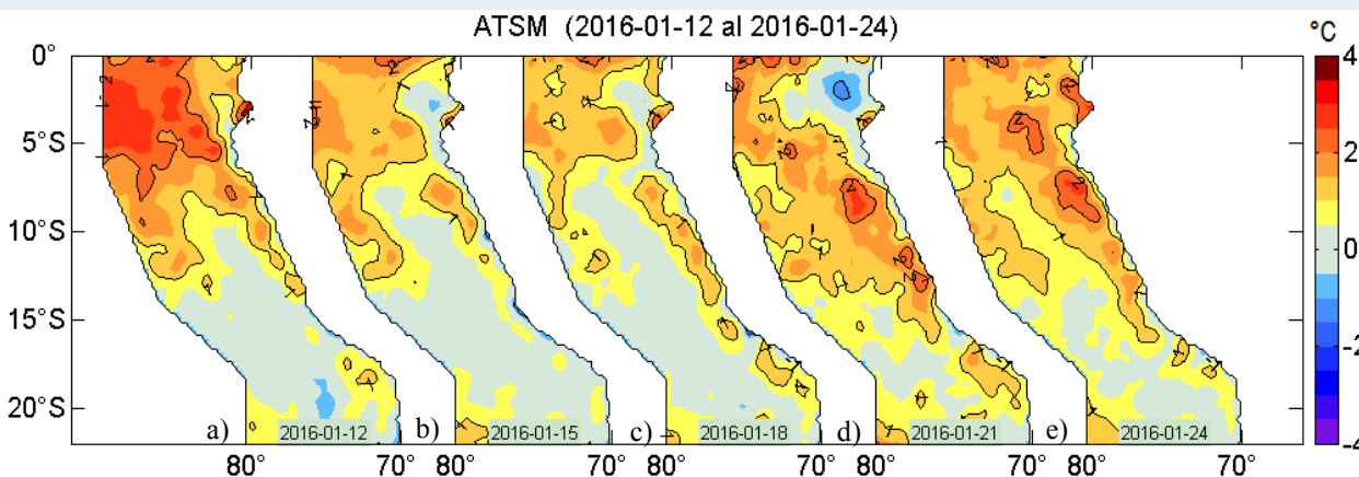
Figura 2. Anomalías de la temperatura superficial del agua (°C) en el mar peruano, cada tres días, entre el 12 al 24 de enero del 2016. Datos: AVHRR/NOAA. Procesamiento: IMARPE.
