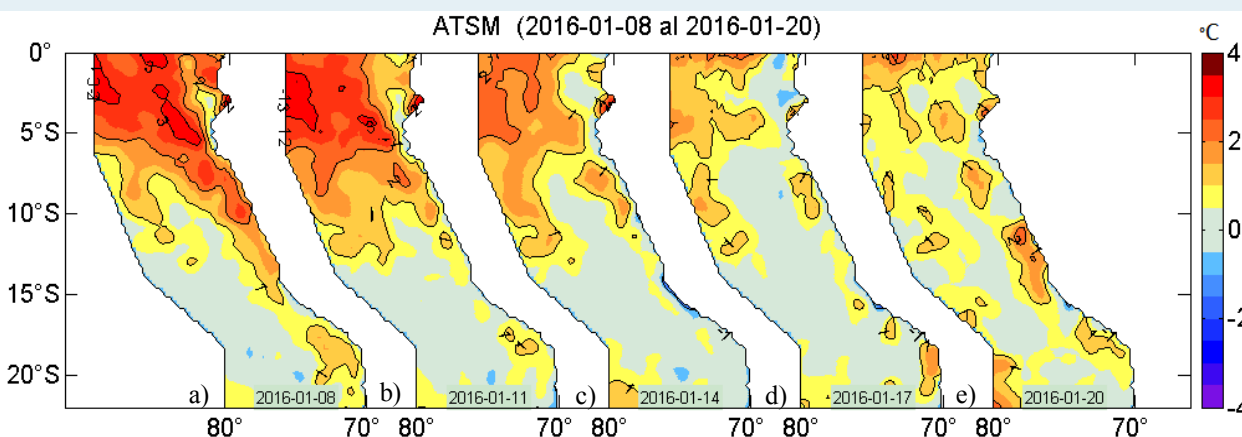
Figura 2. Anomalías de la temperatura superficial del agua (°C) en el mar peruano, cada tres días, entre el 08 y 20 de enero del 2016. Datos: AVHRR/NOAA. Procesamiento: IMARPE.
