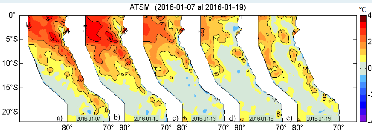
Figura 2. Anomalías de la temperatura superficial del agua (°C) en el mar peruano, cada tres días, entre el 07 y 19 de enero del 2016. Datos: AVHRR/NOAA. Procesamiento: IMARPE.
