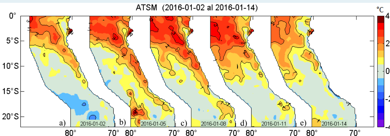
Figura 2. Anomalías de la temperatura superficial del agua (°C) en el mar peruano, cada tres días, del 02 al 14 de enero del 2016. Datos: AVHRR/NOAA. Procesamiento: IMARPE.
