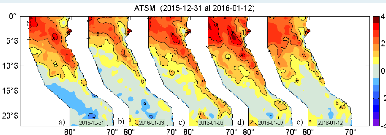
Figura 2. Anomalías de la temperatura superficial del agua (°C) en el mar peruano, cada tres días, entre el 31 de diciembre de 2015 al 12 de enero del 2016. Datos: AVHRR/NOAA. Procesamiento: IMARPE.
