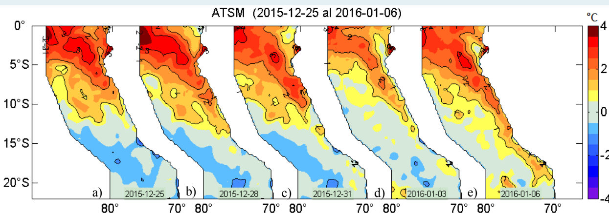
Figura 2. Anomalías de la temperatura superficial del agua (°C) en el mar peruano, cada tres días, entre el 25 de diciembre de 2015 al 6 de enero del 2016. Datos: AVHRR/NOAA. Procesamiento: IMARPE.
