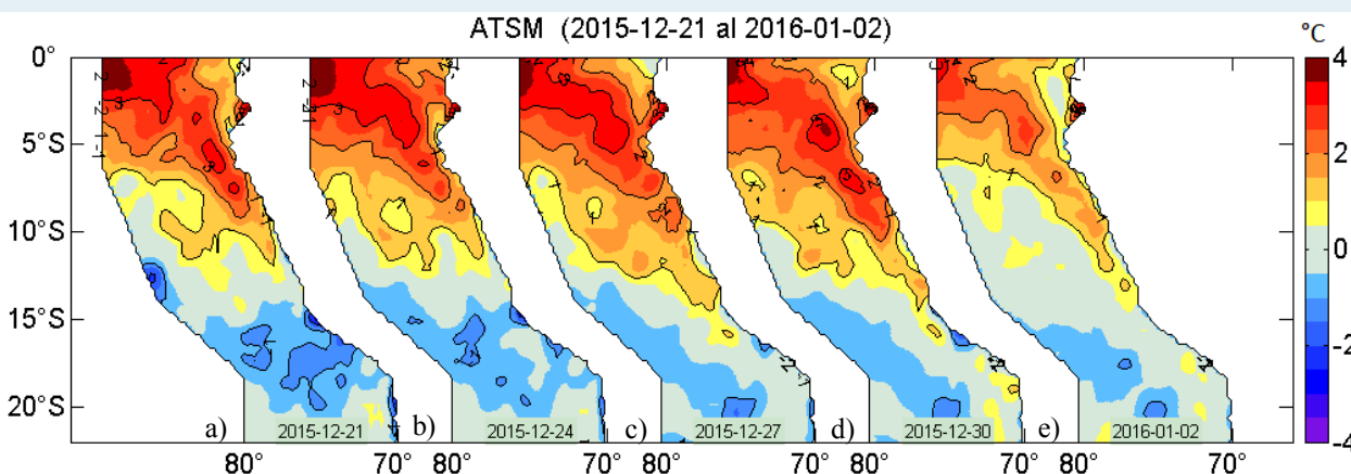
Figura 2. Anomalías de la temperatura superficial del agua (°C) en el mar peruano, cada tres días, entre el 21 de diciembre de 2015 al 2 de enero del 2016. Datos: AVHRR/NOAA. Procesamiento: IMARPE.
