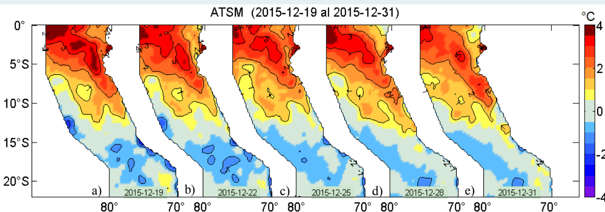
Figura 2. Anomalías de la temperatura superficial del agua (°C) en el mar peruano, cada tres días, entre el 19 y 31 de diciembre de 2015. Datos: AVHRR/NOAA. Procesamiento: IMARPE.
