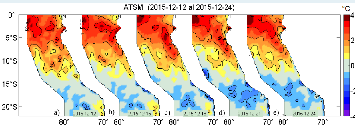
Figura 2. Anomalías de la temperatura superficial del agua (°C) en el mar peruano, cada tres días, entre el 12 y 24 de diciembre de 2015. Datos: AVHRR/NOAA. Procesamiento: IMARPE.
