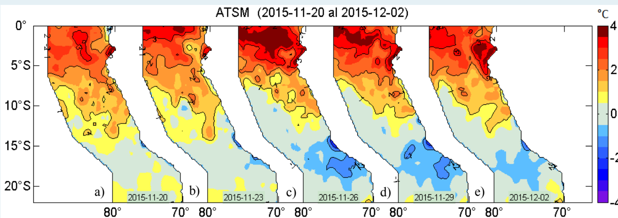
Figura 2. Anomalías de la temperatura superficial del agua (°C) en el mar peruano, cada tres días, entre el 20 de noviembre y 02 de diciembre de 2015. Datos: AVHRR/NOAA. Procesamiento: IMARPE.
