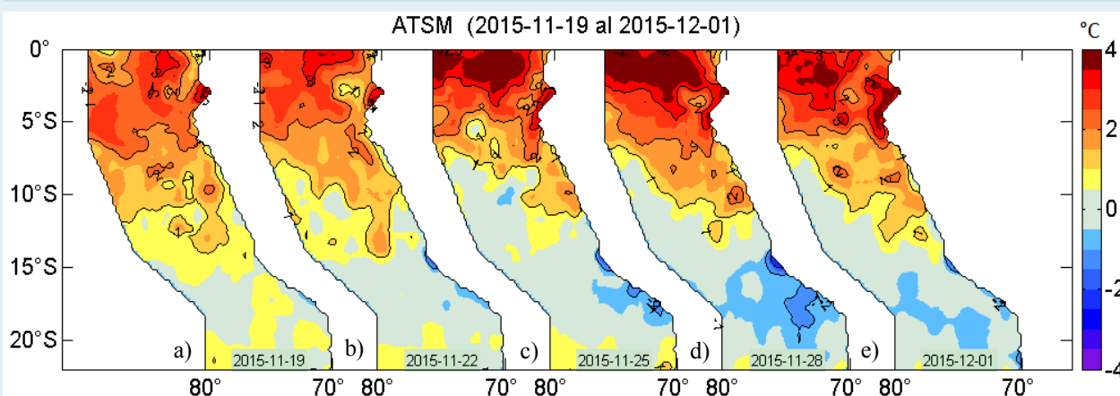
Figura 2. Anomalías de la temperatura superficial del agua (°C) en el mar peruano, cada tres días, entre el 19 de noviembre y 01 de diciembre de 2015. Datos: AVHRR/NOAA. Procesamiento: IMARPE.
