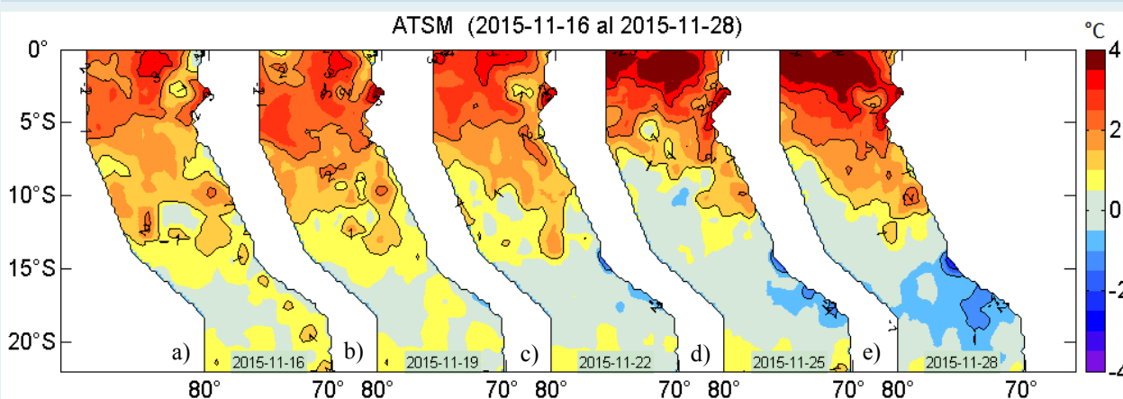
Figura 2. Anomalías de la temperatura superficial del agua (°C) en el mar peruano, cada tres días, entre el 16 al 28 de noviembre de 2015. Datos: AVHRR/NOAA. Procesamiento: IMARPE.
