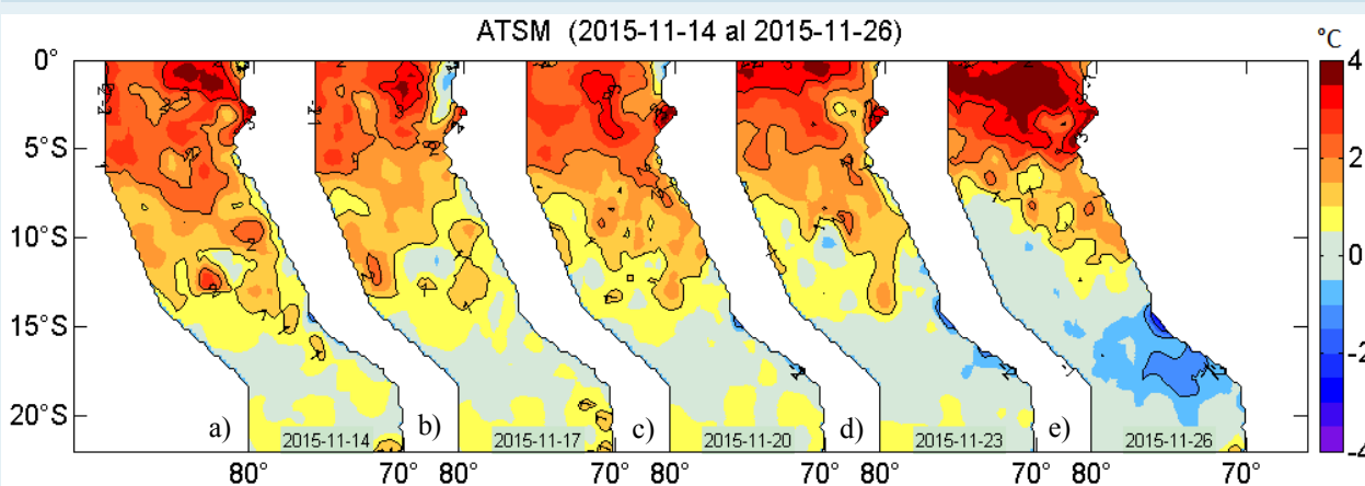
Figura 2. Anomalías de la temperatura superficial del agua (°C) en el mar peruano, cada tres días, entre el 14 al 26 de noviembre de 2015. Datos: AVHRR/NOAA. Procesamiento: IMARPE.
