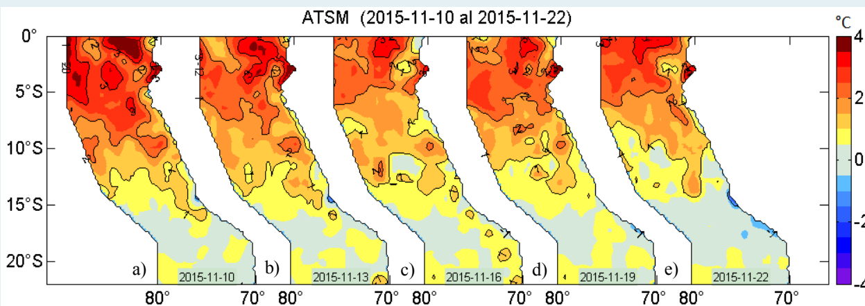
Figura 2. Anomalías de la temperatura superficial del agua (°C) en el mar peruano, cada tres días, entre el 10 al 22 de noviembre de 2015. Datos: AVHRR/NOAA. Procesamiento: IMARPE.
