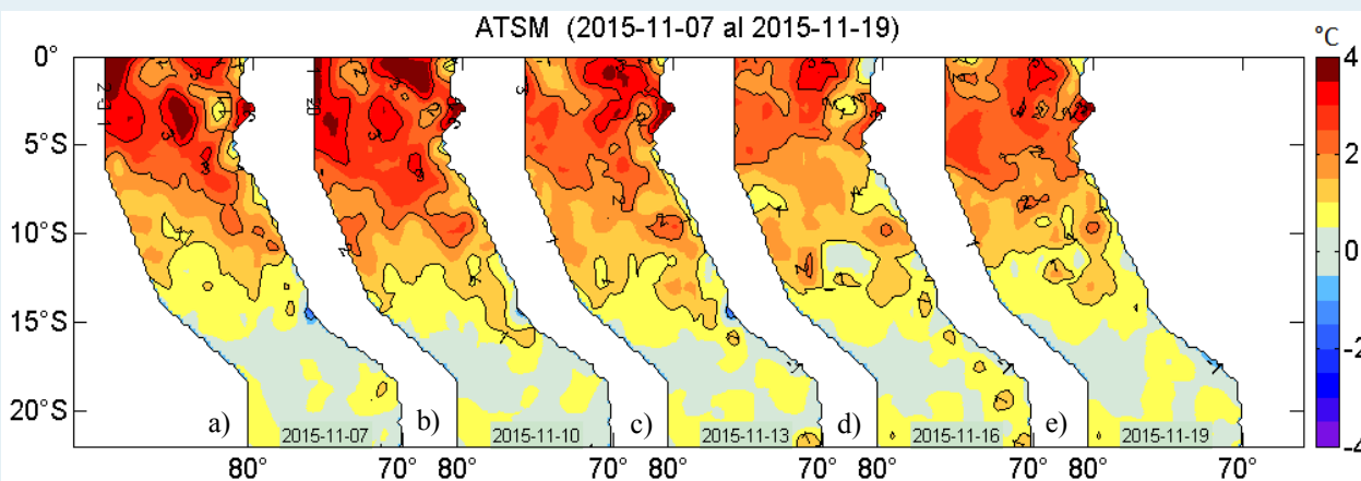
Figura 2. Anomalías de la temperatura superficial del agua (°C) en el mar peruano, cada tres días, entre el 07 al 19 de noviembre de 2015. Datos: AVHRR/NOAA. Procesamiento: IMARPE.
