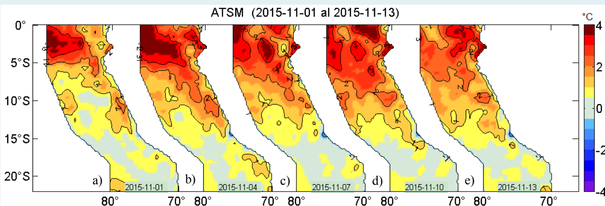
Figura 2. Anomalías de la temperatura superficial del agua (°C) en el mar peruano, cada tres días, entre el 01 al 13 de noviembre de 2015. Datos: AVHRR/NOAA. Procesamiento: IMARPE.
