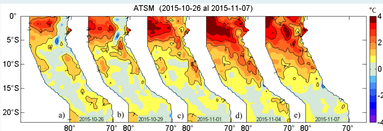
Figura 2. Anomalías de la temperatura superficial del agua (°C) en el mar peruano, cada tres días, entre el 26 de octubre y 07 de noviembre de 2015. Datos: AVHRR/NOAA. Procesamiento: IMARPE.
