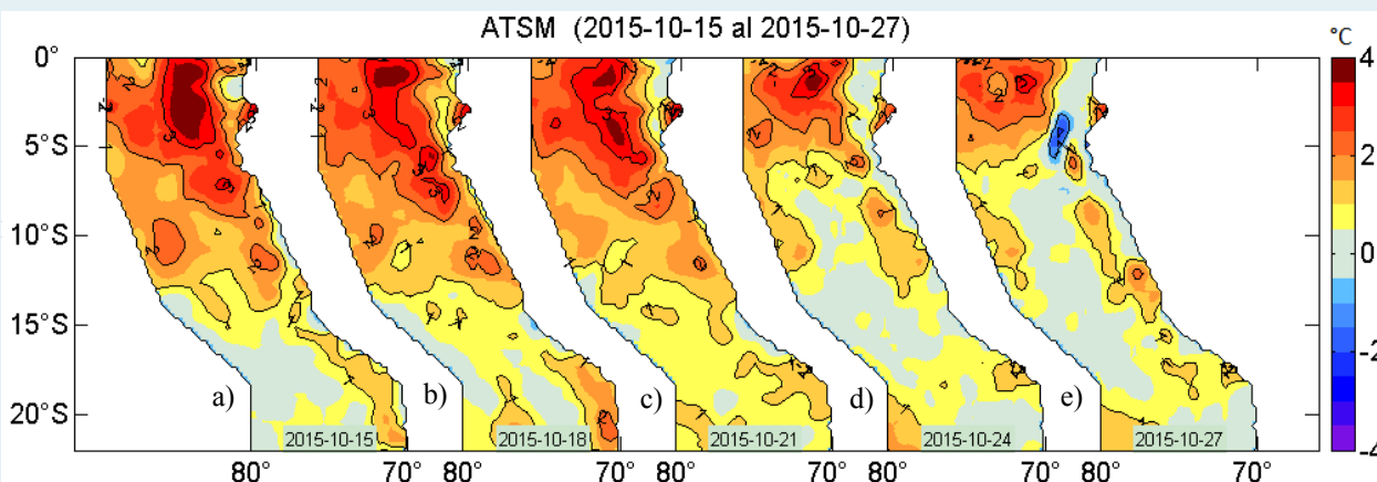
Figura 2. Anomalías de la temperatura superficial del agua (°C) en el mar peruano, cada tres días, del 15 al 27 de octubre de 2015. Datos: AVHRR/NOAA. Procesamiento: IMARPE.
