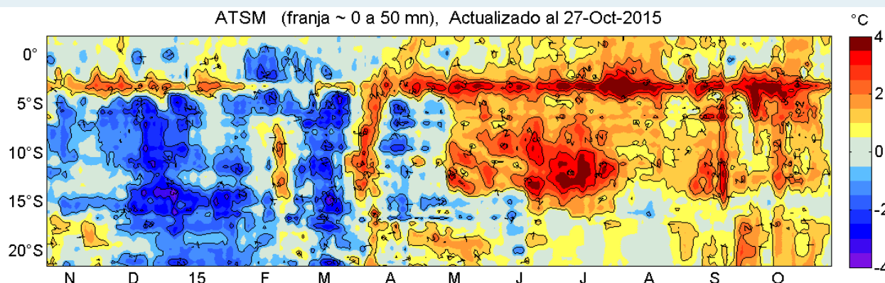
Figura 3. Evolución latitudinal de las anomalías promedio diarias de la temperatura superficial del mar (°C) para la franja de ~50 millas náuticas (mn) adyacentes al litoral peruano. Datos: AVHRR/NOAA. Procesamiento: IMARPE.
