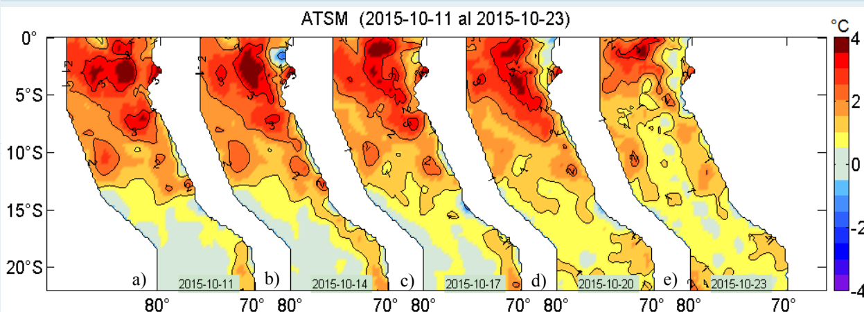
Figura 2. Anomalías de la temperatura superficial del agua (°C) en el mar peruano, cada tres días, entre el 11 y 23 de octubre de 2015. Datos: AVHRR/NOAA. Procesamiento: IMARPE.
