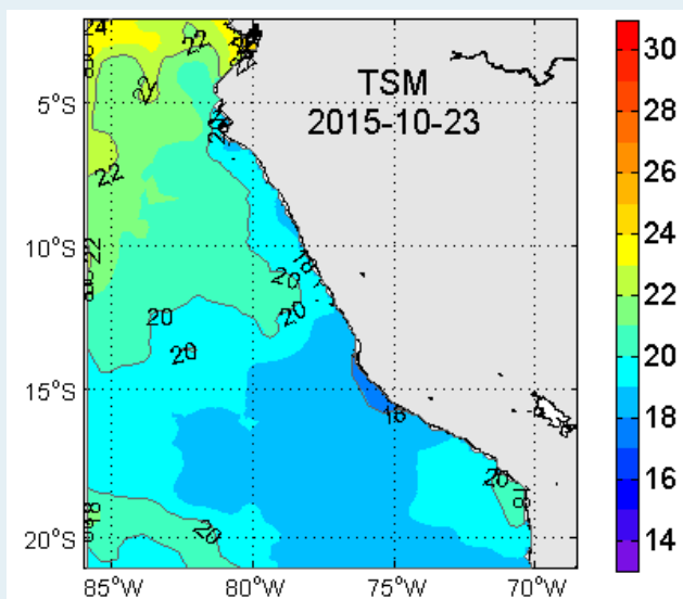
Figura 4. Distribución espacial de la temperatura superficial del mar peruano (°C). Datos: AVHRR/NOAA. Procesamiento: IMARPE.
