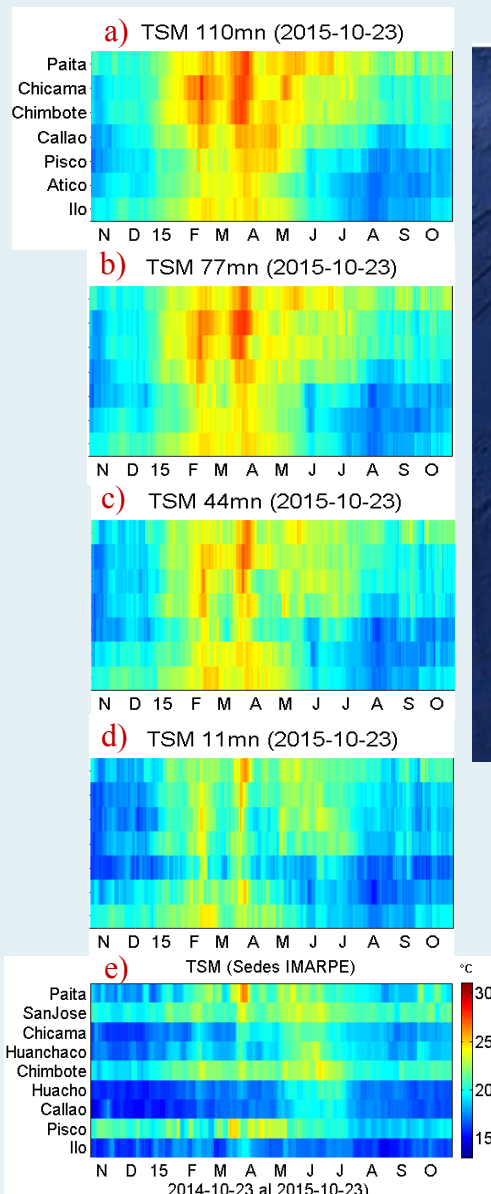
Figura 4. Distribución espacial de la temperatura superficial del mar peruano (°C). Datos: AVHRR/NOAA. Procesamiento: IMARPE.
