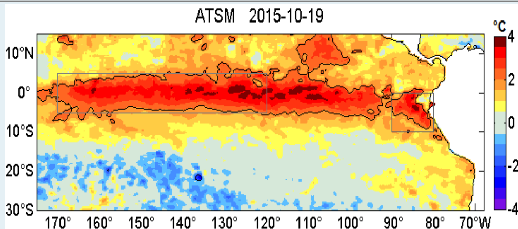
Figura 1. Anomalías de la temperatura superficial del mar (°C) en el océano Pacífico tropical. Las regiones Niño 3.4 y Niño 1+2 en los sectores central y oriental del océano, respectivamente, están delimitadas con una línea delgada de color negro. Datos: AVHRR/NOAA. Procesamiento: IMARPE.
