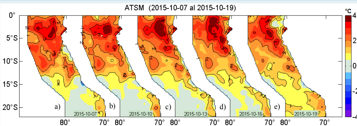
Figura 2. Anomalías de la temperatura superficial del agua (°C) en el mar peruano, cada tres días, entre el 07 y 19 de octubre de 2015. Datos: AVHRR/NOAA. Procesamiento: IMARPE.
