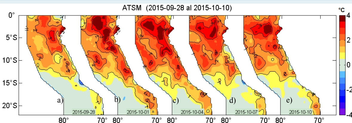
Figura 2. Anomalías de la temperatura superficial del agua (°C) en el mar peruano cada tres días entre el 28 de setiembre y 10 de octubre. Datos: AVHRR/NOAA. Procesamiento: IMARPE.
