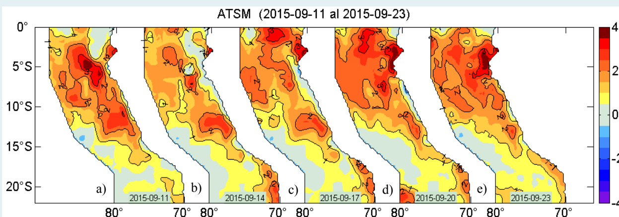
Figura 2. Anomalías de la temperatura superficial del agua ( ^{\circ}\text{C} ) en el mar peruano los días a) 11, b) 14, c) 17, d) 20, y e) 23 de setiembre. Datos: AVHRR/NOAA. Procesamiento: IMARPE.
