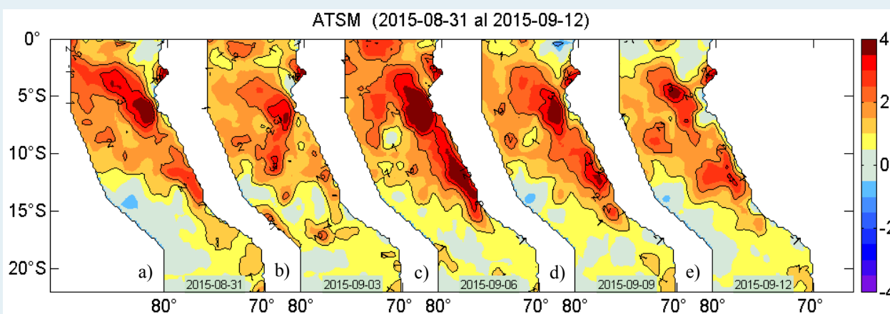
Figura 2. Anomalías de la temperatura superficial del agua (°C) en el mar peruano los días a) 31 de agosto, b) 03 de setiembre, c) 06 de setiembre, d) 09 de setiembre, y e) 12 de setiembre. Datos: AVHRR/NOAA. Procesamiento: IMARPE.
