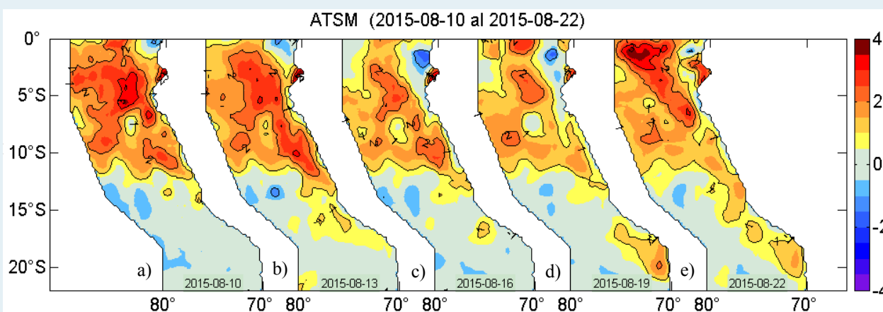
Figura 2. Anomalías de la temperatura superficial del agua ( ^{\circ}\text{C} ) en el mar peruano los días a) 10, b) 13, c) 16, d) 19, y e) 22 de agosto. Datos: AVHRR/NOAA. Procesamiento: IMARPE.
