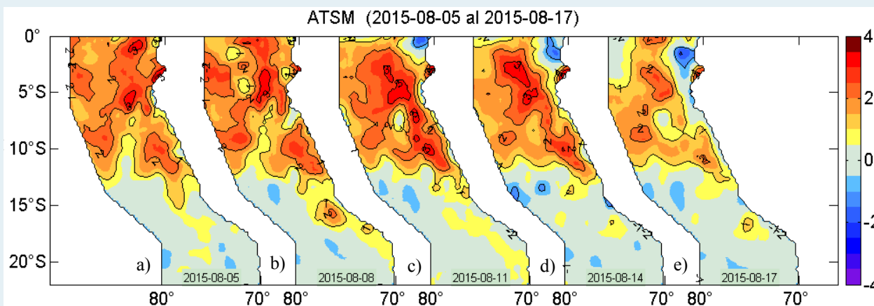
Figura 2. Anomalías de la temperatura superficial del agua (°C) en el mar peruano los días a) 05, b) 08, c) 11, d) 14, y e) 17 de agosto. Datos: AVHRR/NOAA. Procesamiento: IMARPE.
