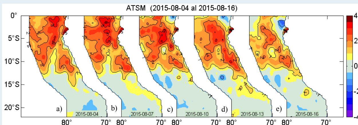
Figura 2. Anomalías de la temperatura superficial del agua (°C) en el mar peruano los días a) 04, b) 07, c) 10, d) 13, y e) 16 de agosto. Datos: AVHRR/NOAA. Procesamiento: IMARPE.
