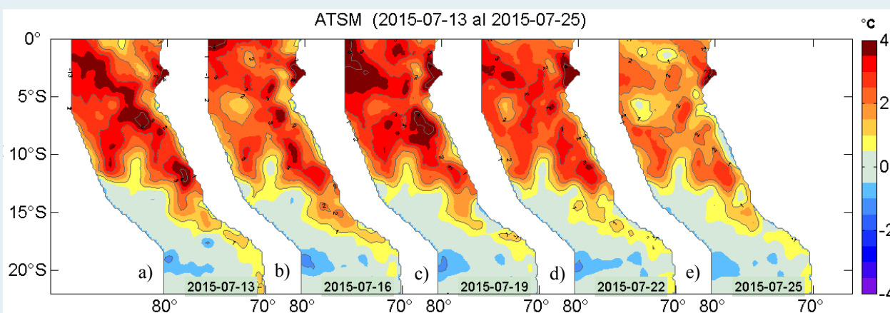
Figura 2. Anomalías de la temperatura superficial del agua (°C) en el mar peruano los días a) 13, b) 16, c) 19, d) 22 y e) 25 de julio. Datos: AVHRR/NOAA. Procesamiento: IMARPE.
