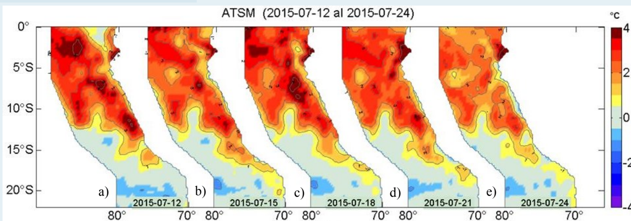
Figura 2. Anomalías de la temperatura superficial del agua (°C) en el mar peruano los días a) 12, b) 15, c) 18, d) 21 y e) 24 de julio. Datos: AVHRR/NOAA. Procesamiento: IMARPE.
