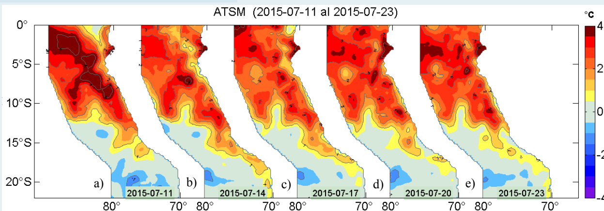
Figura 2. Anomalías de la temperatura superficial del agua ( ^{\circ}\text{C} ) en el mar peruano los días a) 11, b) 14, c) 17, d) 20 y e) 23 de julio. Datos: AVHRR/NOAA. Procesamiento: IMARPE.
